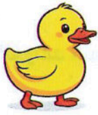
duck بطة
