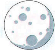
moon قمر
