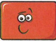
rectangle مستطيل
